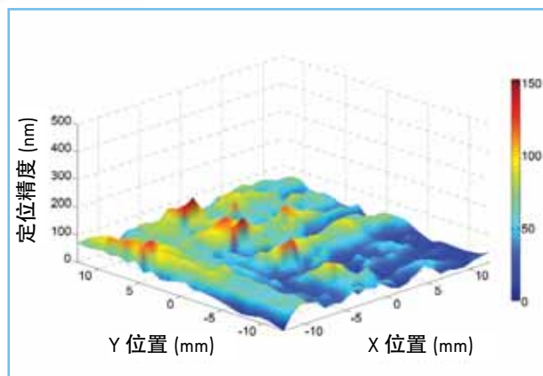
ANT95-XY 版本 2D 定位精度
