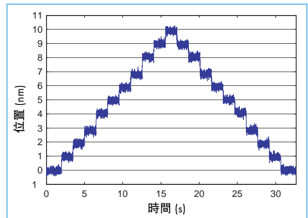
ANT130-060-L-PLUS 1 nm 步階圖
